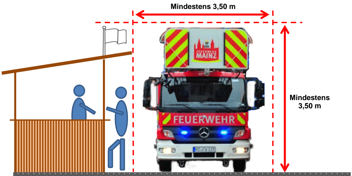
Abb. 2: Mindestdurchfahrtsbreite und -höhe
